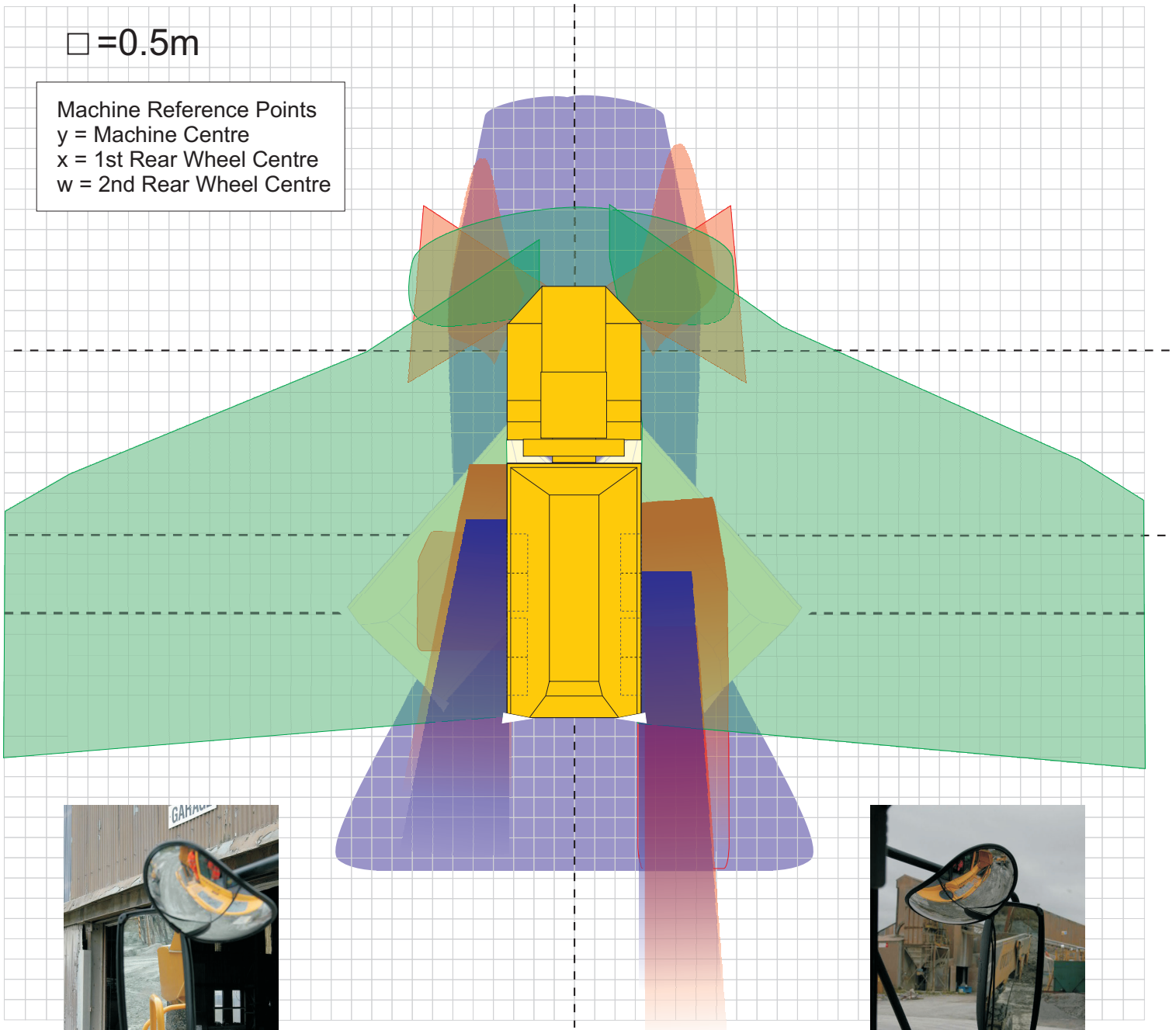
Volvo A35
