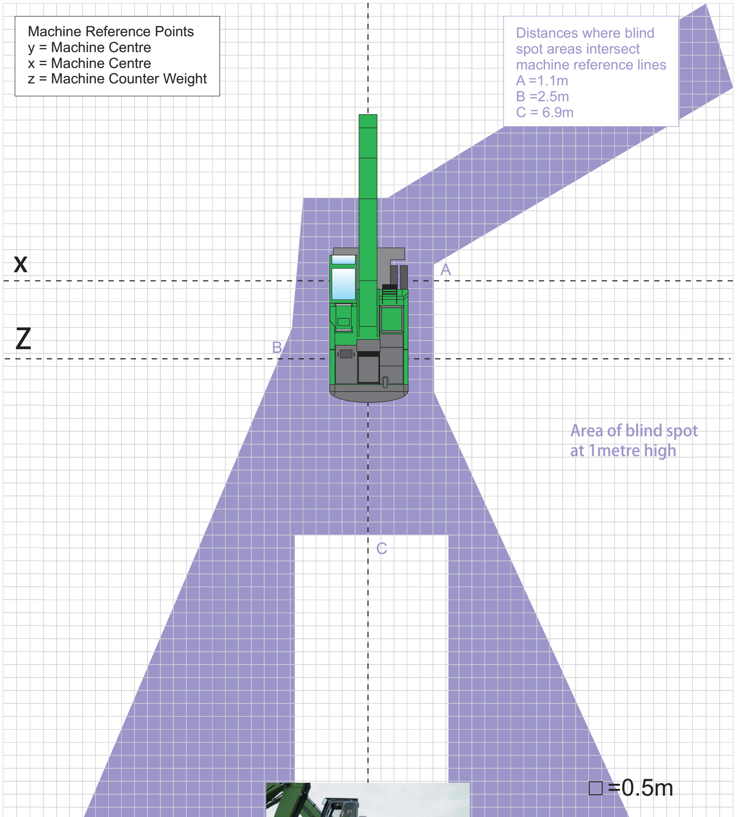
Sennebogen 830M
