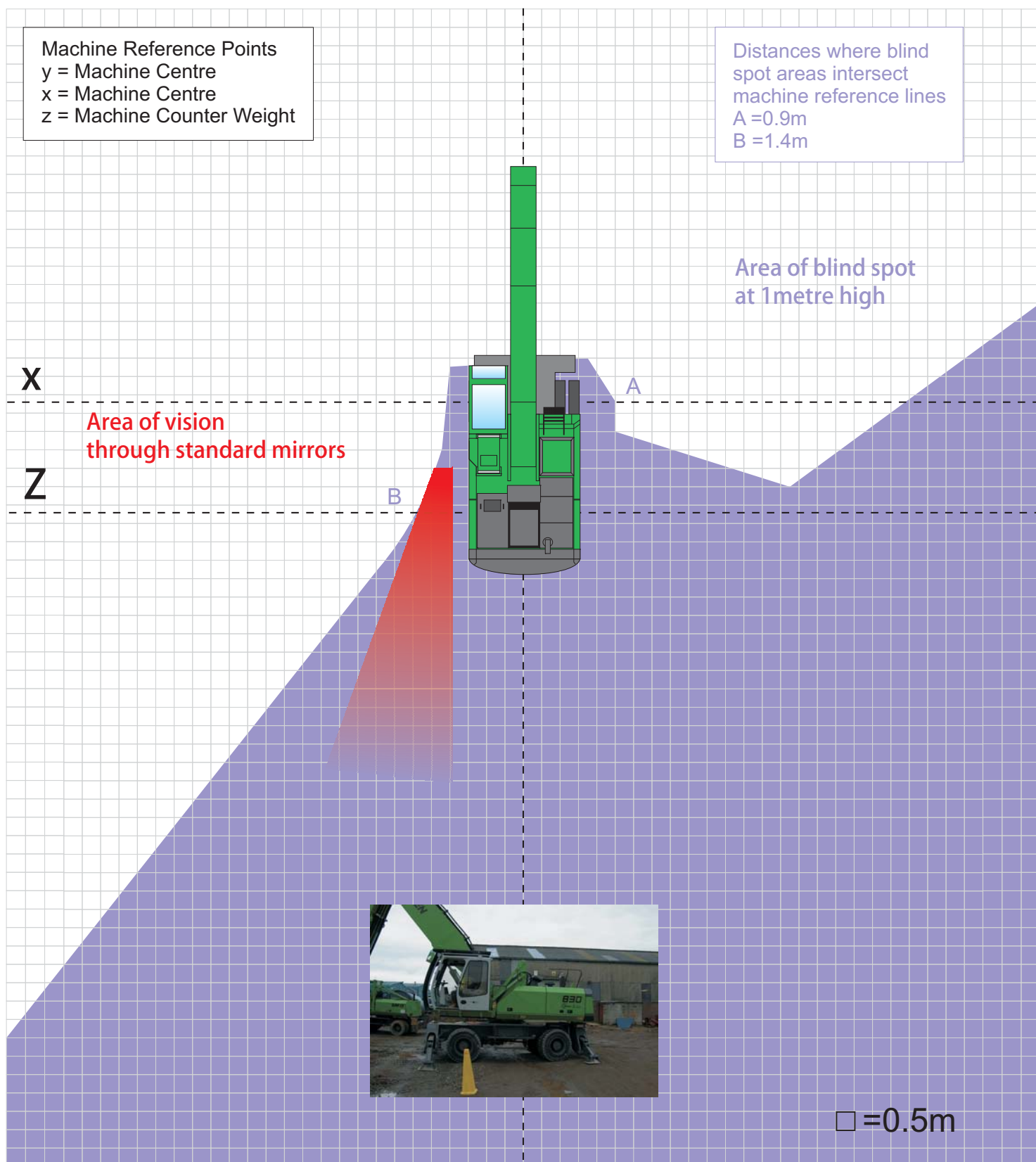
Sennebogen 830M
