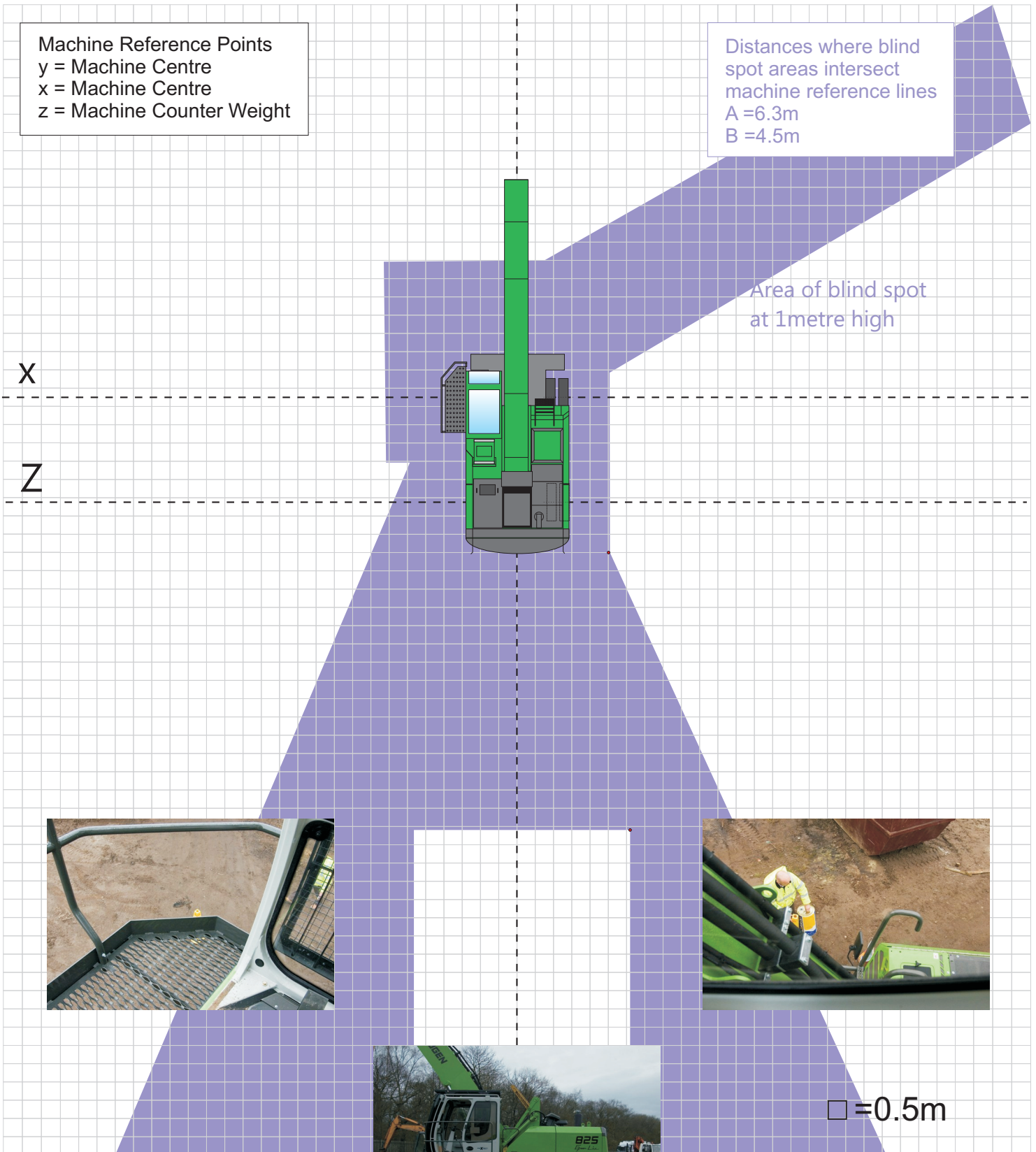
Sennebogen 825M
