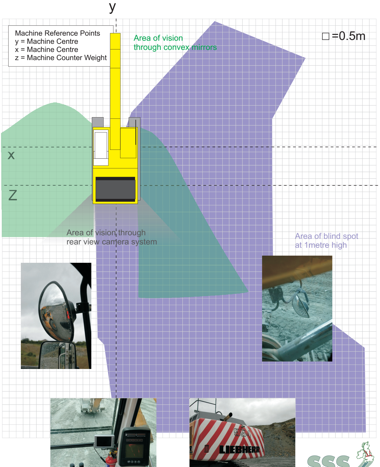
Liebherr 954
