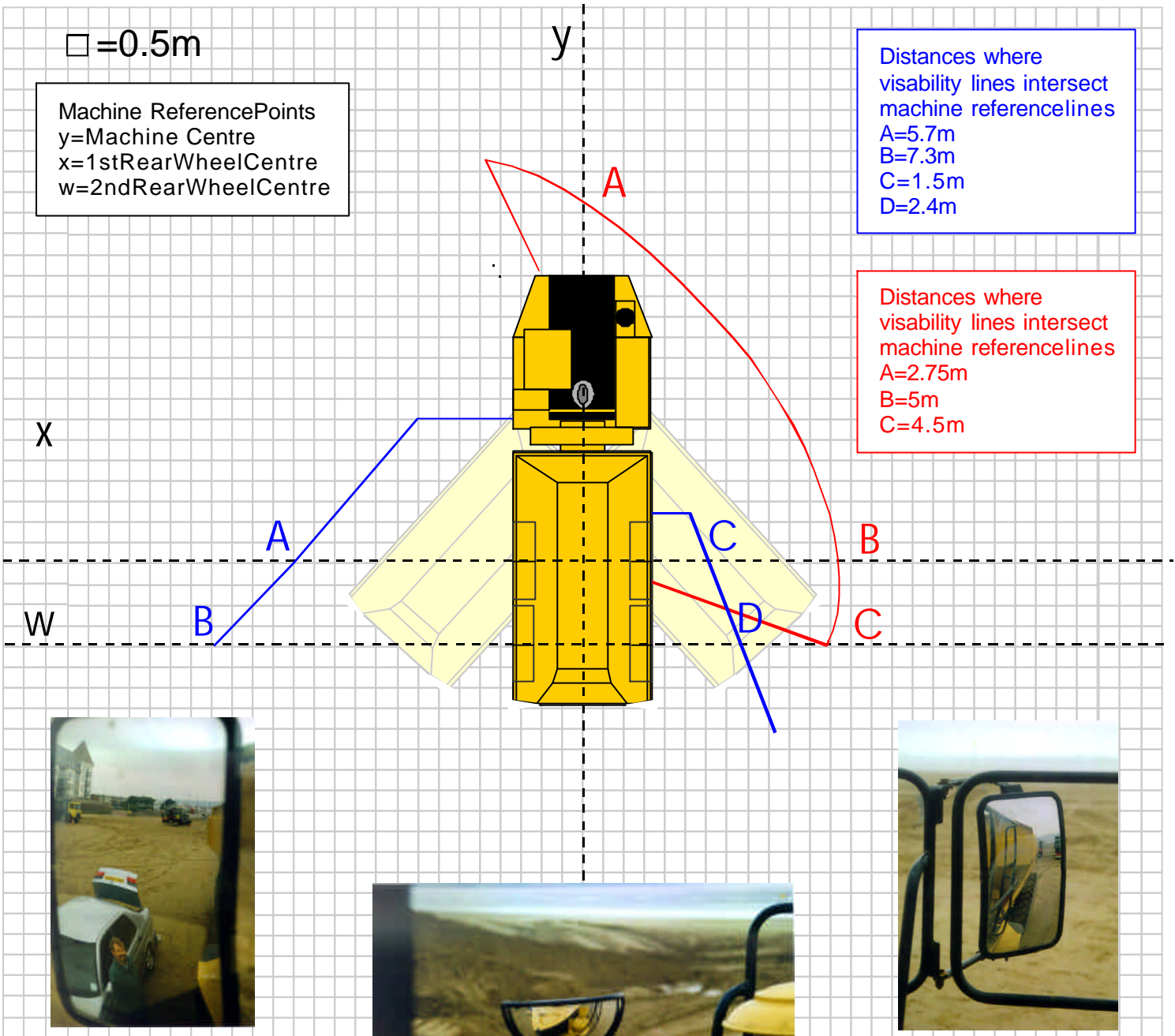
CAT D400E
