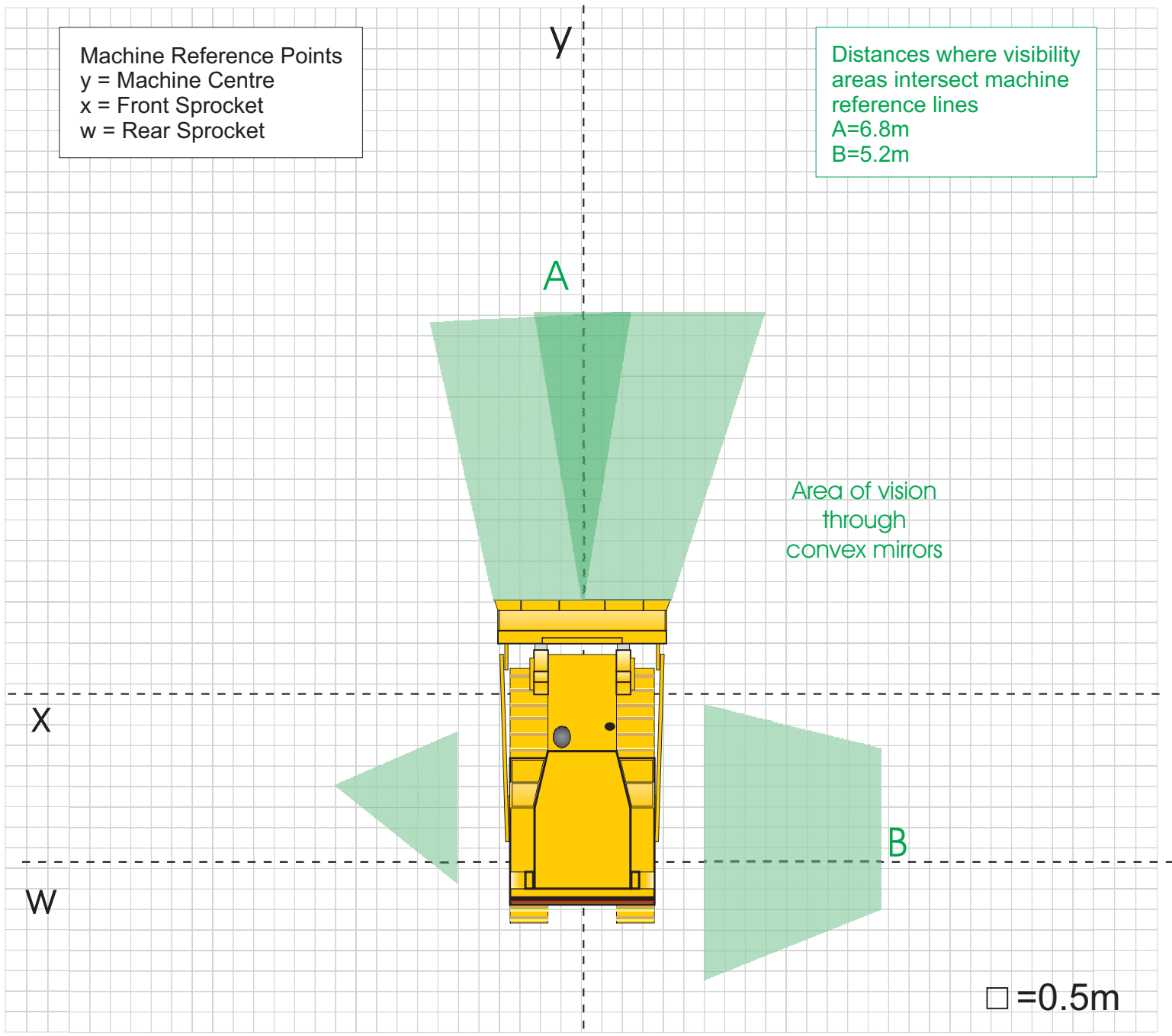
CAT D10R
