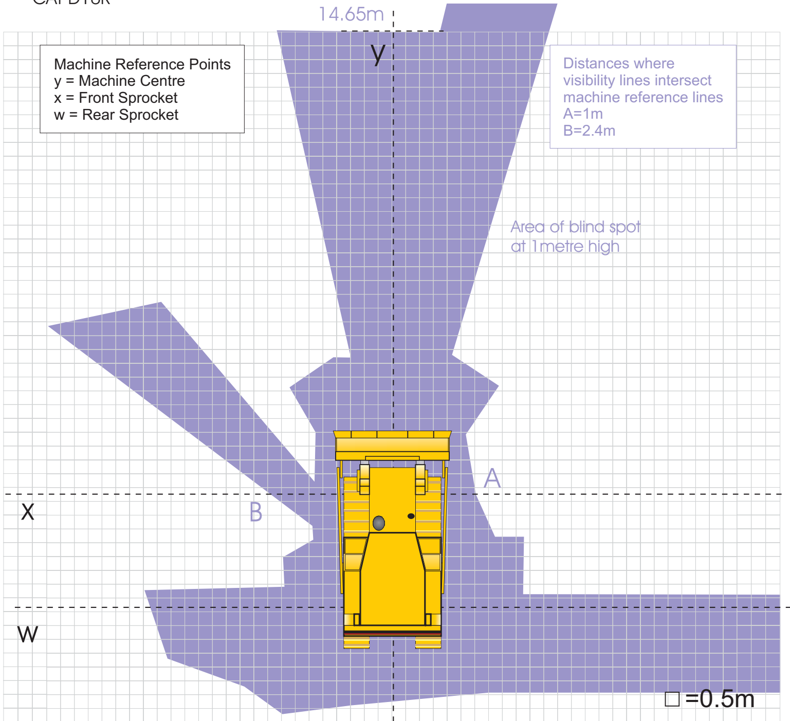
CAT D10R
