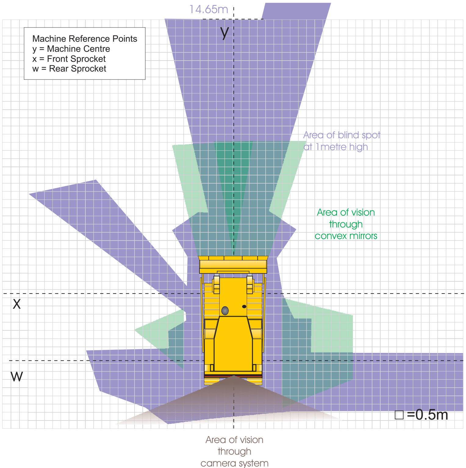
CAT D10R
