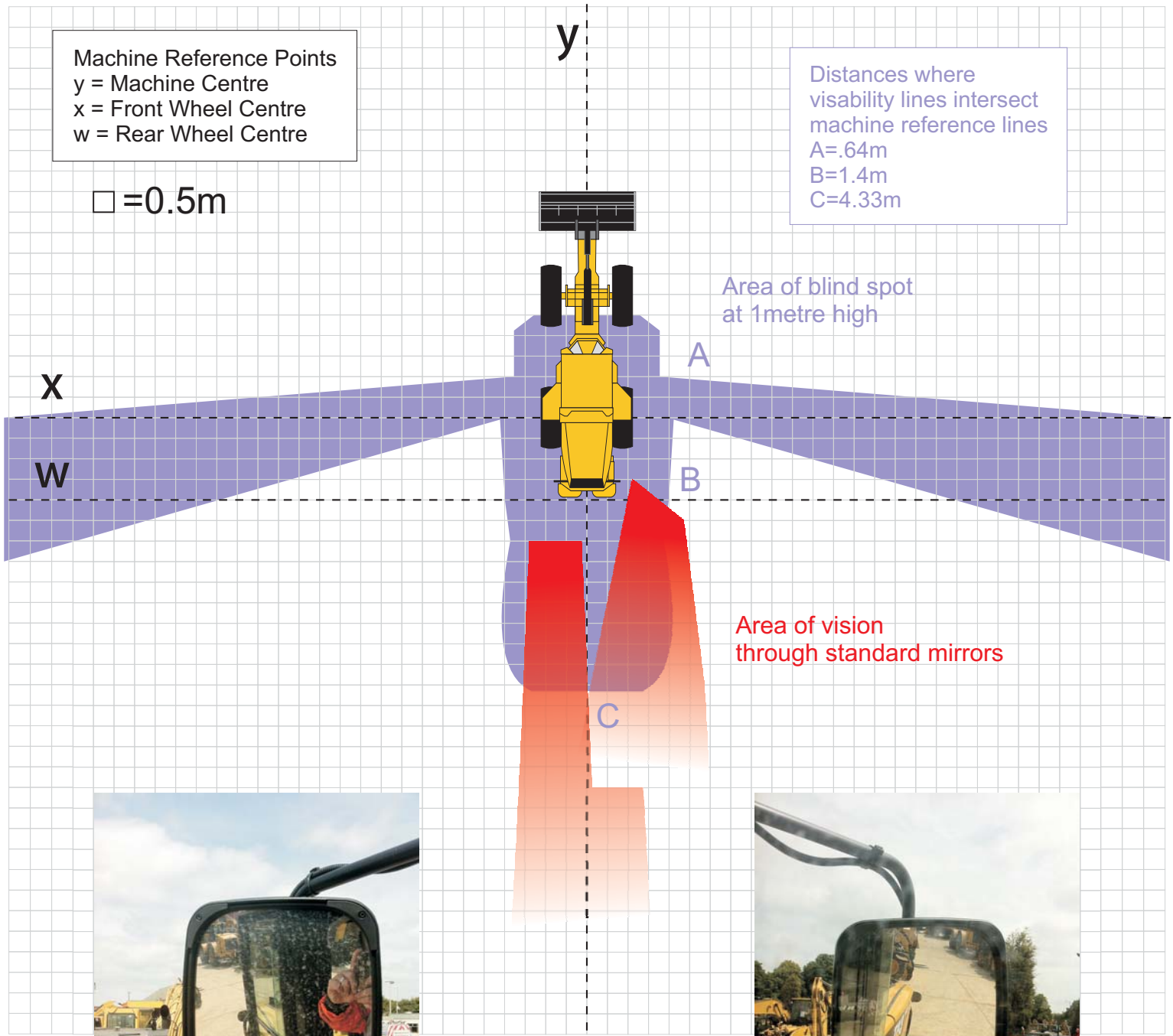
CAT 930H
