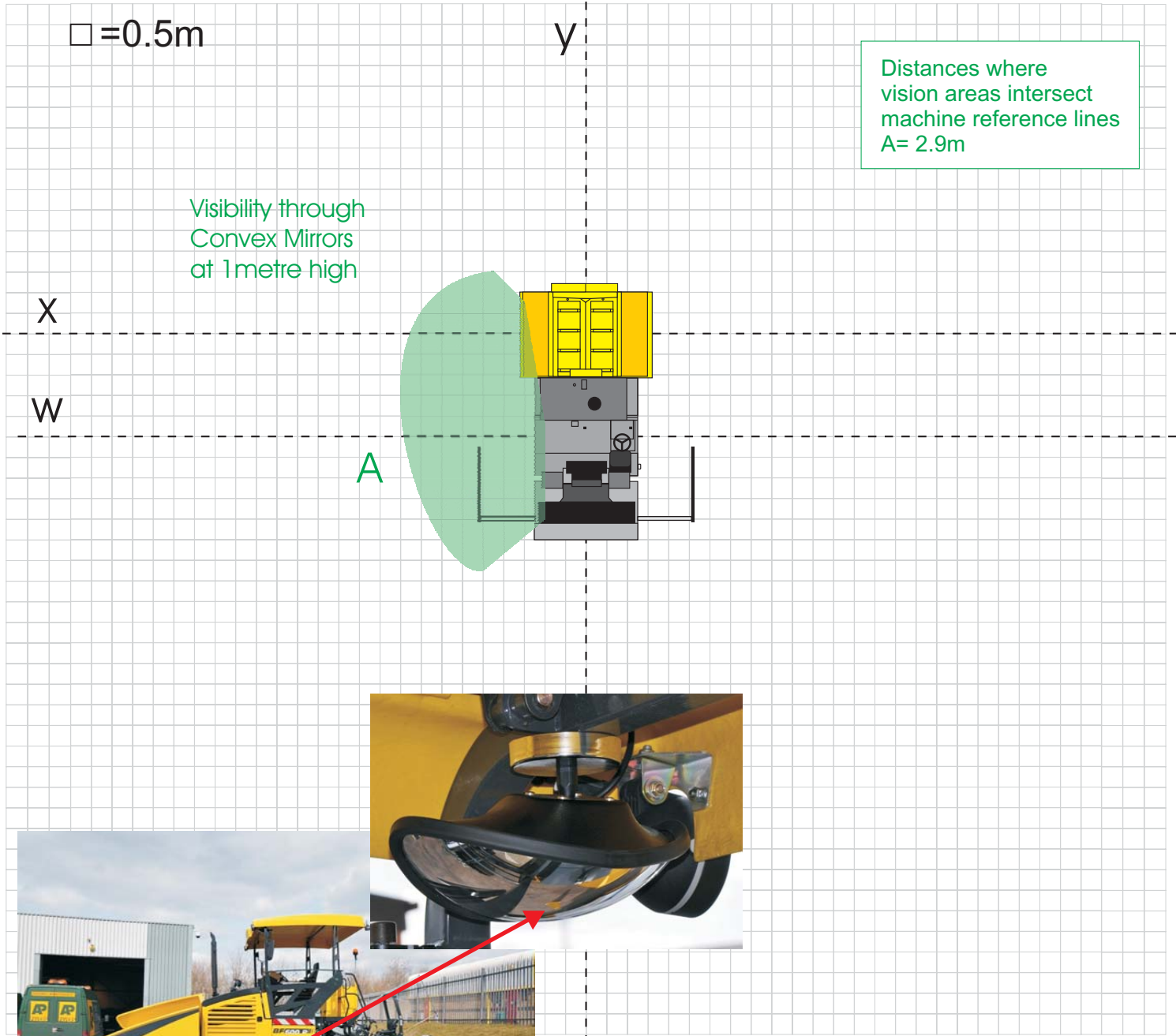
Bomag BF 600
