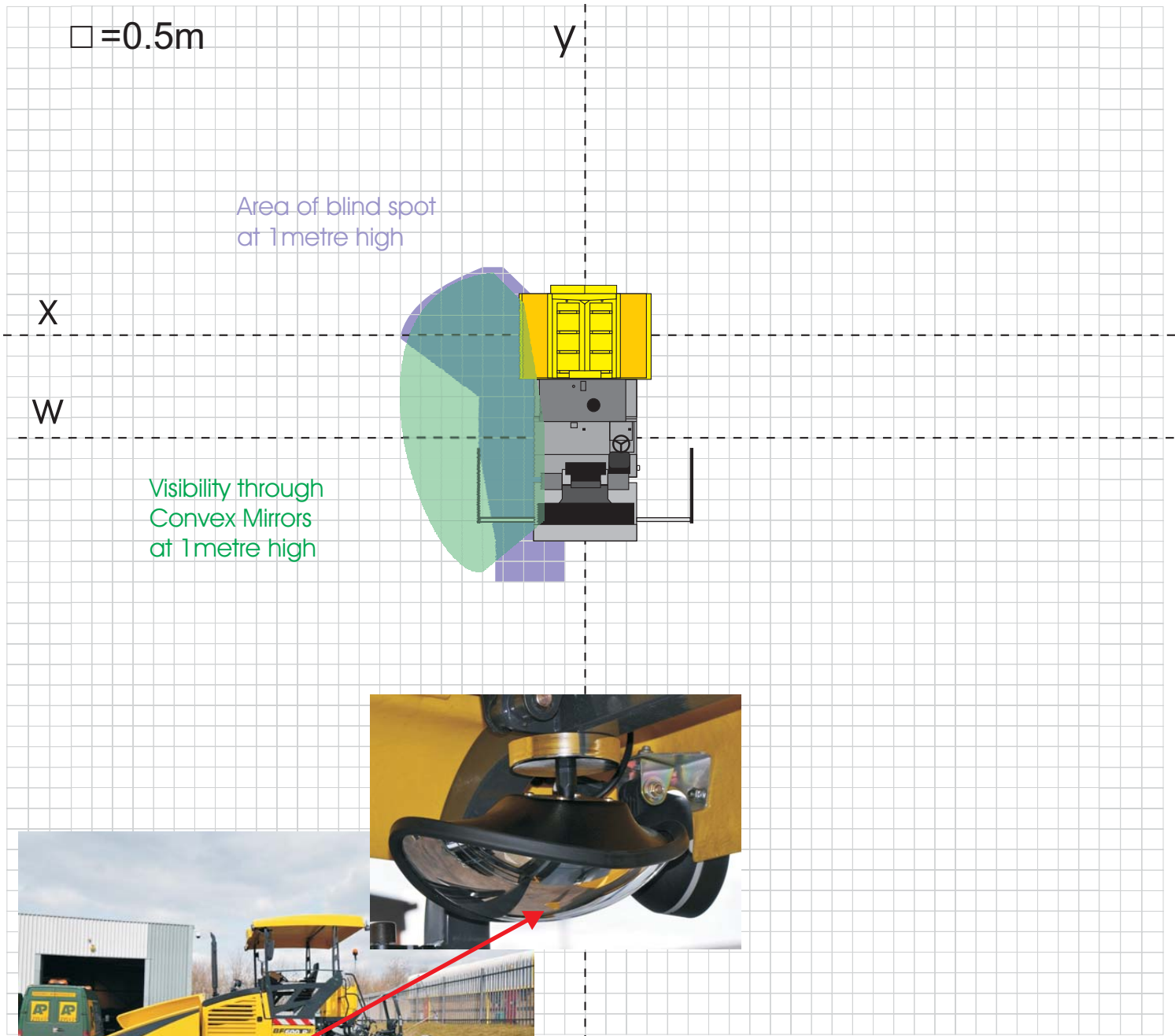
Bomag BF 600
