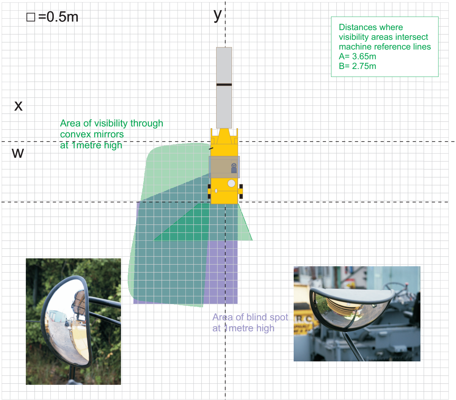
Bitelli SF102R
