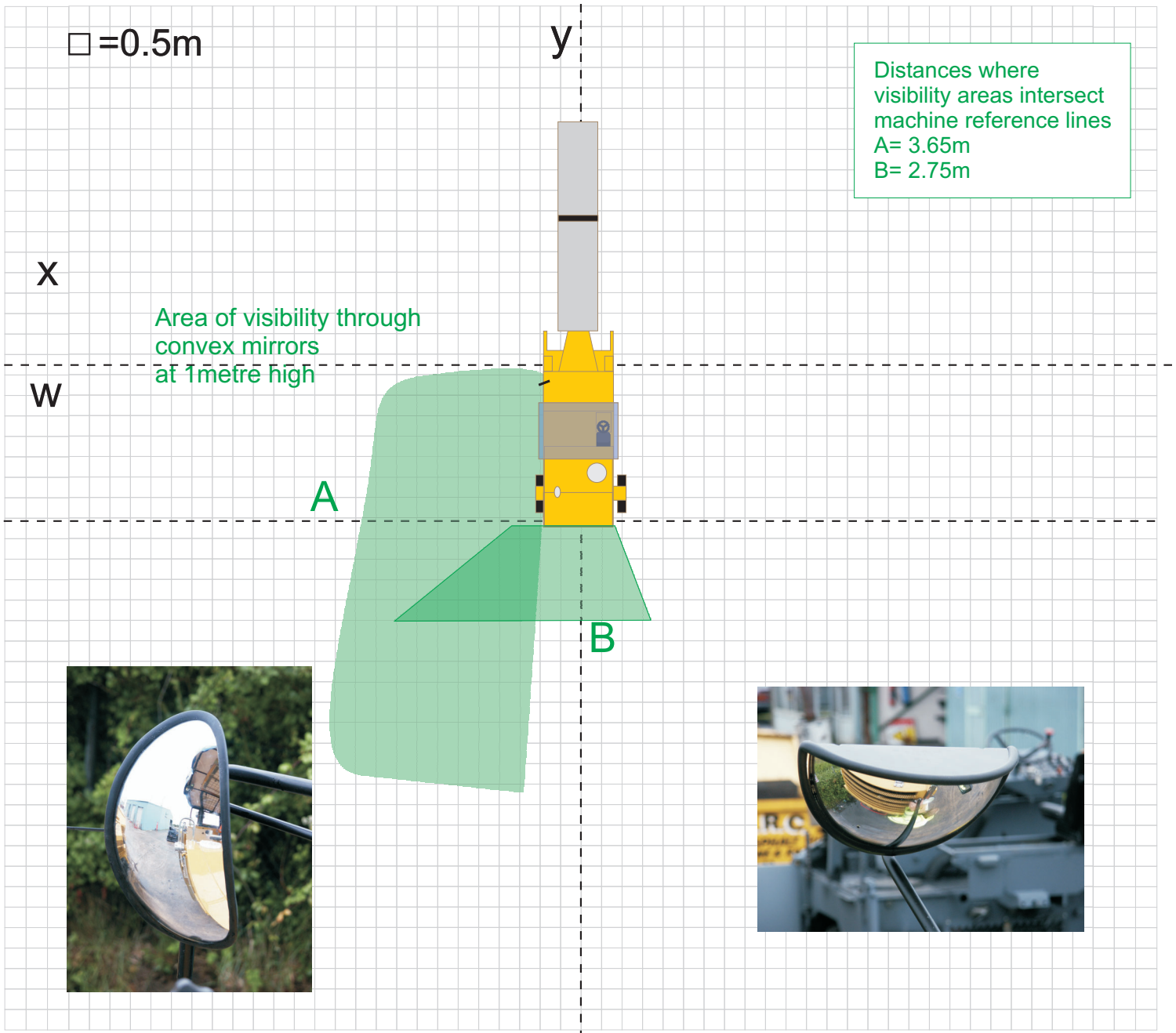
Bitelli SF102R
