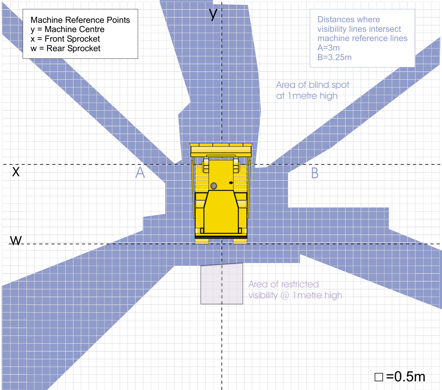
CAT D9T
