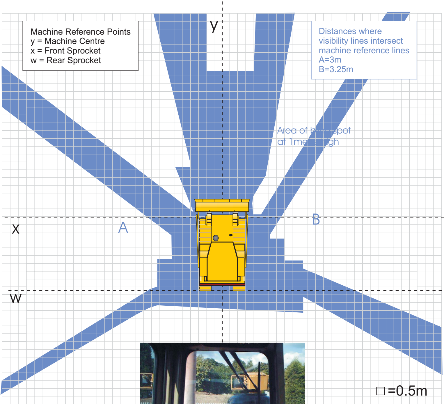
CAT D9R
